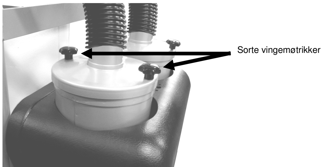
Figur 4 Toppen af HEPA filterholderen på en ME2800
