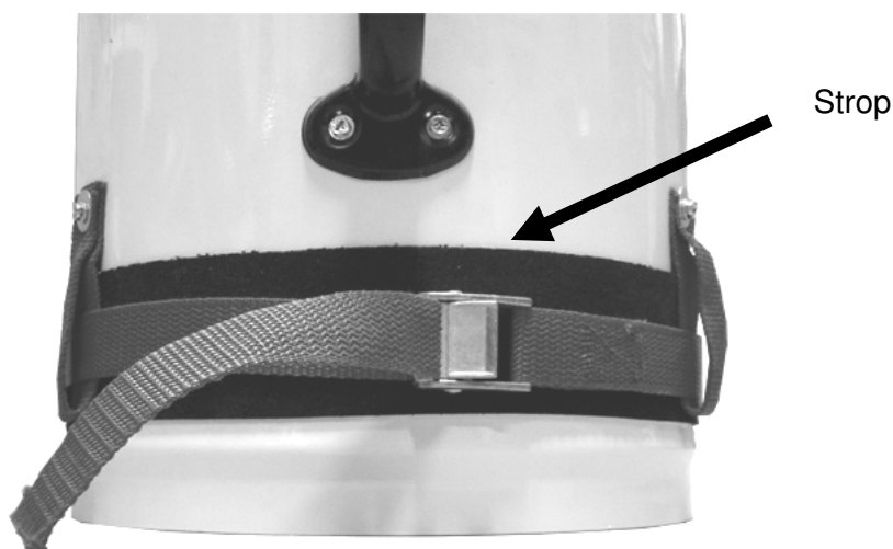
Figur 2 Holder til opsamlingspose
