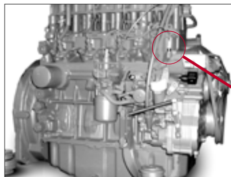
Fig. - 85 Motortempera- turføler
