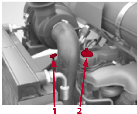
Fig. - 75 Kontrol af motoroliestand / påfyldning af olie
