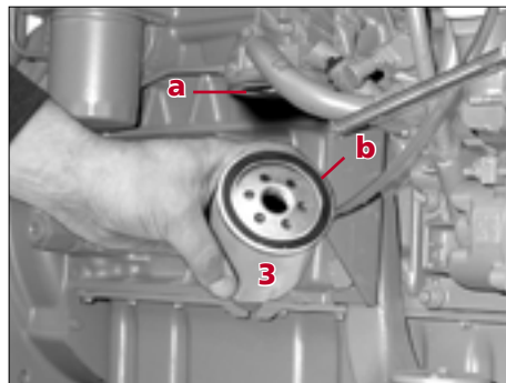
Fig. - 80 Brændstof-hovedfilter
