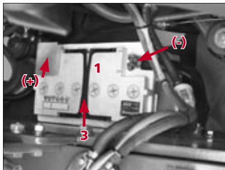
Fig. - 101 Batteriets placering
