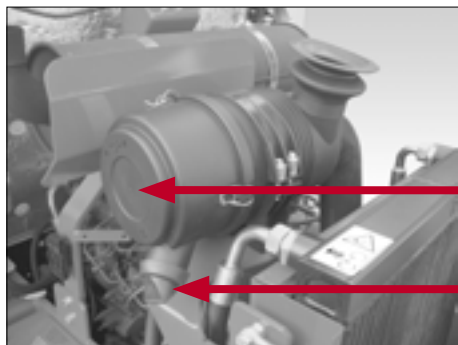
Fig. - 82 Luftfilterets placering
