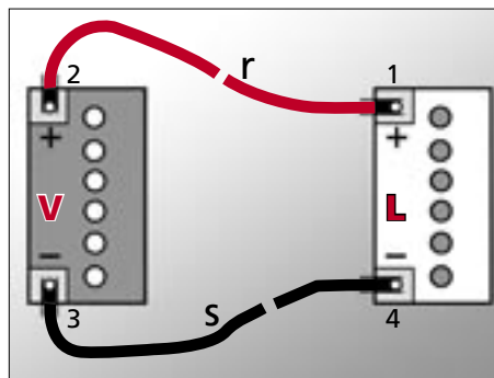
Fig. - 102 Tilslutning af startkabler
