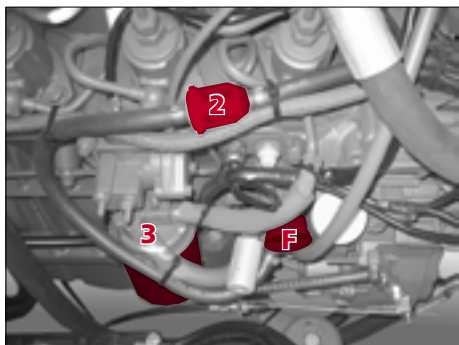
Fig. - 78 Brændstoffilterets position
