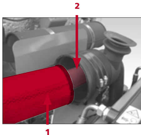
Fig. - 83 Luftfilter-ele- menter
