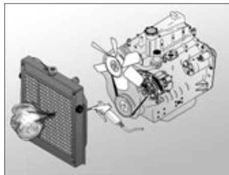
Fig. - 89 Rengøring af kølesystemet
