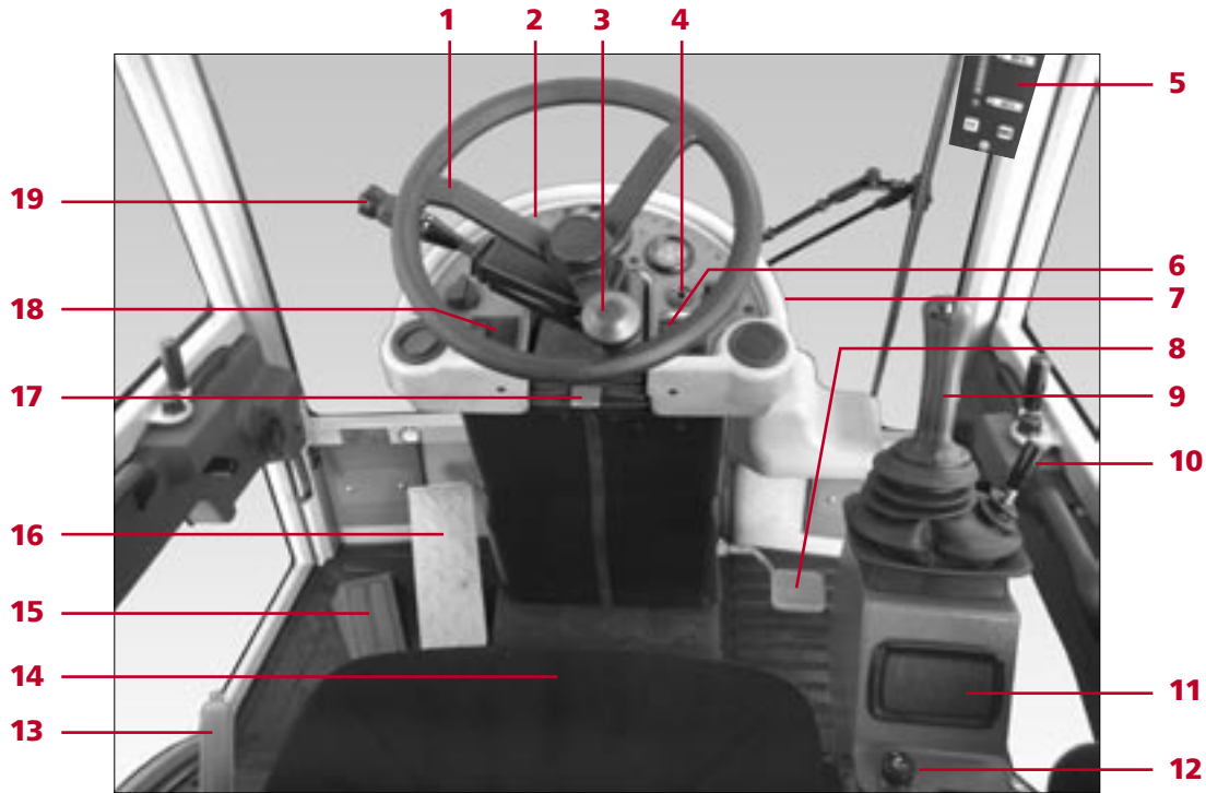
Fig. - 13 Betjeningsselementer
