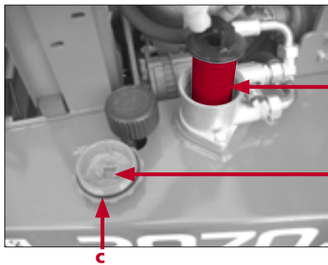
Fig. - 95 Filterindsats
