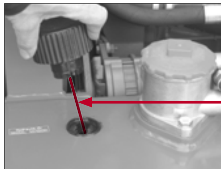
Fig. - 92 Målepind til hydraulisk olie
