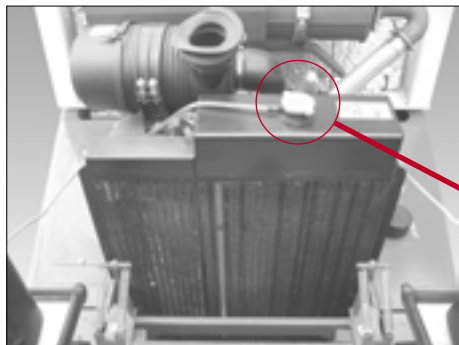
Fig. - 87 Køleråbning (Perkins-motor)
