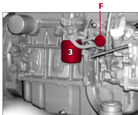
Fig. - 79 Brændstoffilterets position Deutz-motor
