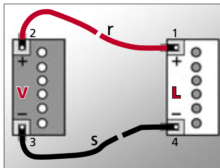
Fig. - 105 Tilslutning af startkabler
