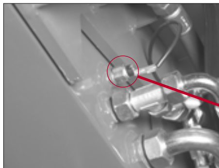
Fig. - 85 Hydraulisk olie- temperaturføler
