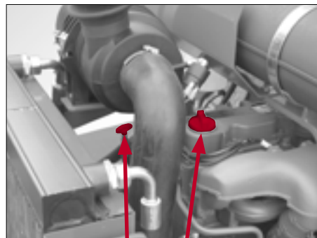
Fig. - 76 Kontrol af motoroliestand / påfyldning af olie
