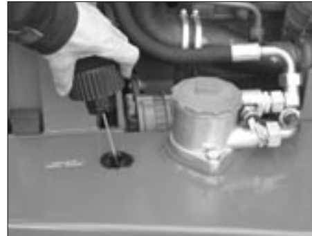
Fig. - 67 Reducering af resttrykket
