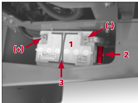
Fig. - 104 Batteriets placering
